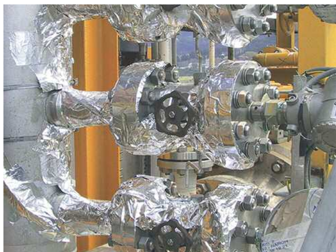
Cubrimiento del traceado con aislamiento
