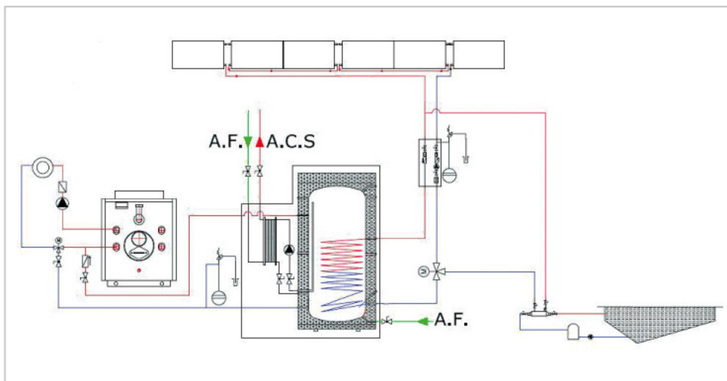
Esquema instalación solar térmica
